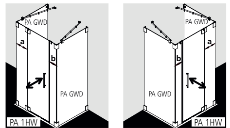
U-Kabine: PA 1HW und PA GWD und PA GWD
