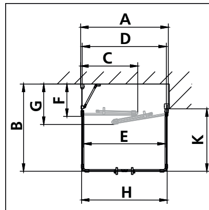
Maßanfertigung Schacht- / Fensteranbindung
