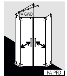
U-Kabine: PA PFD und PA GWD (Seite 165)
