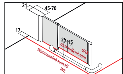
Breitenverstellmaß BV = Wanneneinbaumaß WE - 10
