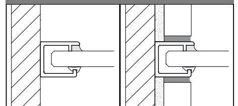
Optionales Wandprofil für Befestigung ohne Beschläge (siehe Zubehör Seite 226).
