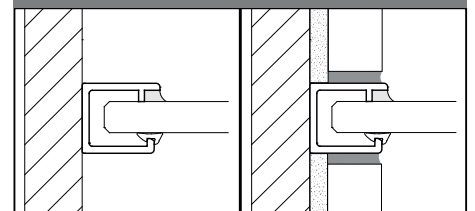
Optionales Wandprofil für Befestigung ohne Beschläge (siehe Zubehör Seite 284)
