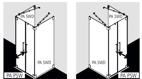
U-Kabine: PA PSW und PA SWD und PA SWD
